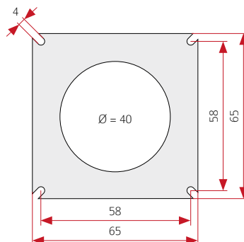
Lautsprecher (Einbautiefe: 26 mm)
